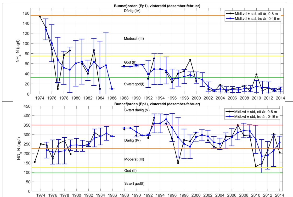
Figur 29. Vinterobservasjoner av \text{NH}_4\text{-N} (øverste panel) og \text{NO}_3\text{-N}+\text{NO}_2\text{-N} (nederste panel) i Bunnfjorden (Ep1). For detaljert forklaring, se i Figur 26
