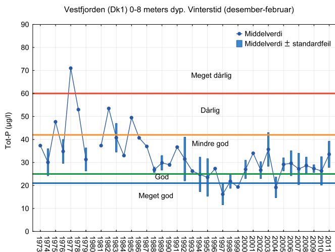
Figur 3. Vinterobservasjoner av Tot-P i Vestfjorden (Dk1) i 0, 4 og 8 meters dyp for perioden 1973-2011. Det er først beregnet middelværdi over dyp for hver dato, deretter er gjennomsnitt over datoene innenfor hver vinterperiode beregnet. Årstall gjelder månedene januar og februar, men hver vinterperiode omfatter også data fra desember året før. Mengden av data bak hvert gjennomsnitt vil variere noe fra år til år. Verdiene fra enkelte år kan avvike sterkt som følge av lokale flommer, varierende grad av algeoppblomstring, eller varierende tidspunkt for dypvannsfornyelse. De høyere konsentrasjonene i 2003 er eksempelvis dypere "gammelt" vann som ble løftet opp til overflaten ved en vannfornyelse. Utviklingen er sammenlignet med Klima- og forurensningsdirektoratet (Klif) sitt miljøklassifiseringssystem for vannkvalitet. I perioden 1970-1985 var tilstanden ofte dårlig/meget dårlig. Siden da har det skjedd en klar bedring; de siste 20 år har tilstanden stort sett variert fra meget god/god til mindre god.
