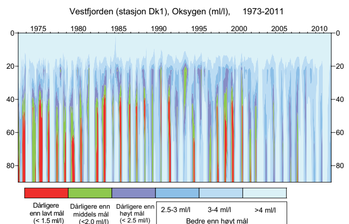
Figur 8. Oksygenkonsentrasjonen i Vestfjorden (Dk1) 1973-2011, sammenlignet med tentative miljømål. Bare variasjon under 4 ml/l er markert i figuren. Oksygenkonsentrasjonen i dyplagene har blitt bedre siden 1970-tallet og har siden 2008 hatt konsentrasjoner omkring høyt mål.
